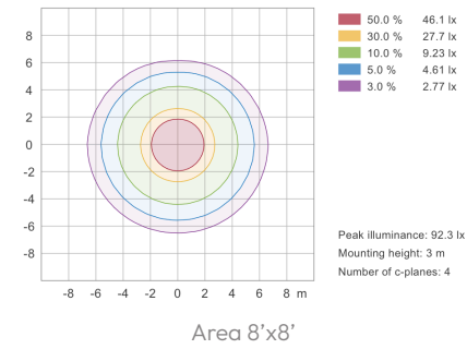
Iso-illuminance plot
