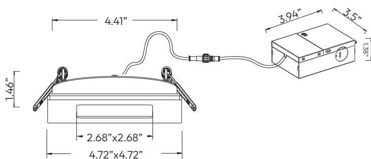
Technical Drawing: 4.41" (D) x 4.72" (W) x 1.46" (H)
