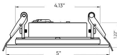
Technical Drawing: 5" (D) x 4.13" (W) x 1.22" (H)
