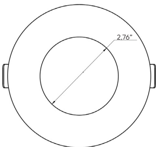
Technical Drawing: 5" (D) x 4.13" (W) x 1.22" (H)
